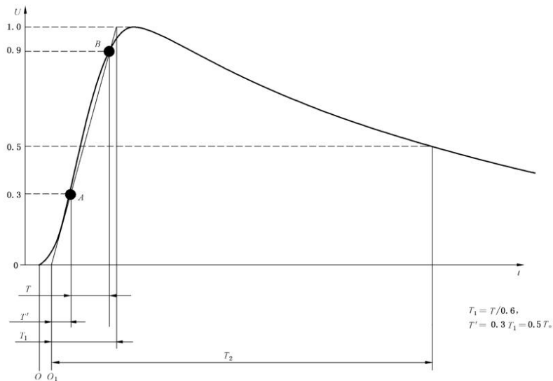
图 1 试验装置冲击电压波形时间参数的确定
