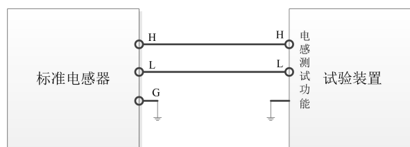
图 10a 三端接线方式电感校准试验装置接线图
