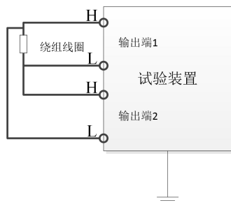
图 8a 两组交替输出型试验装置波形面积校准接线图
