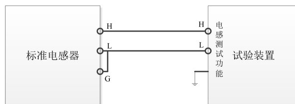
图 10b 二端接线方式电感校准试验装置接线图
