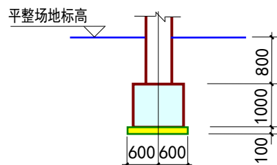
二-8 题图 某条形基础断面示意
