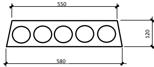
三-5 题图 某空心板断面示意图
