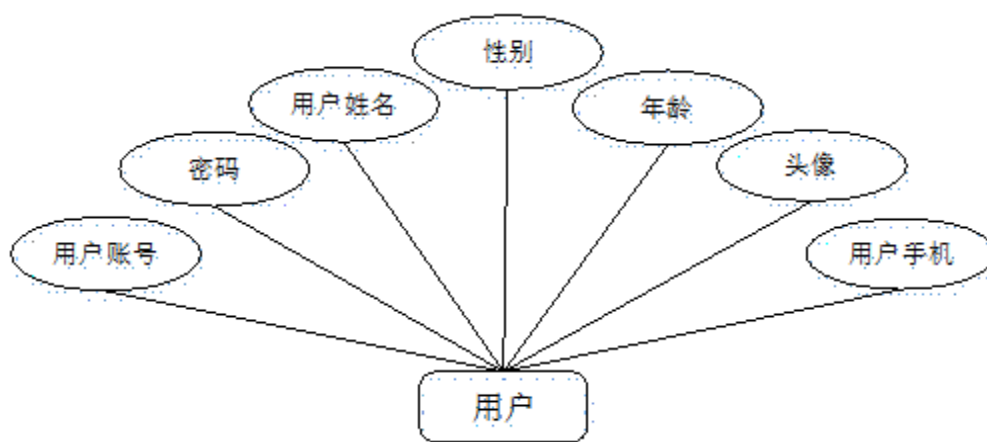
图 4-3 用户 E/R 图
