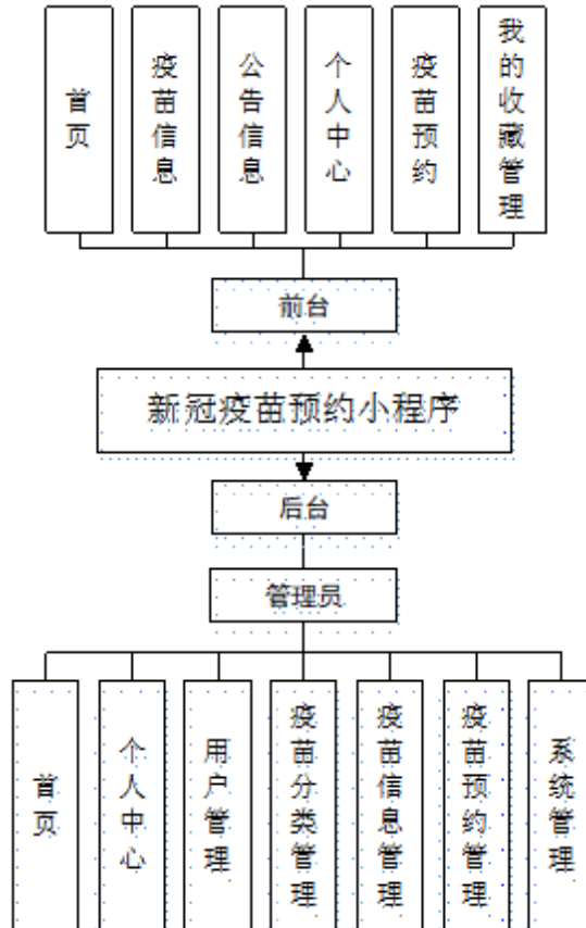
图 4-1 小程序总体结构图
