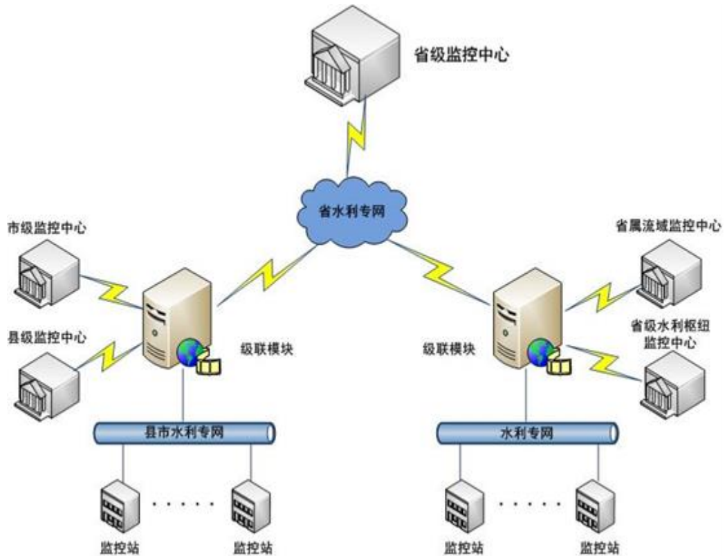
图 4-1 系统总体拓扑图
