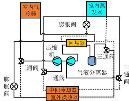
(b)中间冷却式 \text{CO}_2 热泵
