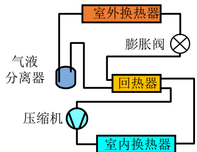
(a)带回热器的 \text{CO}_2 热泵
