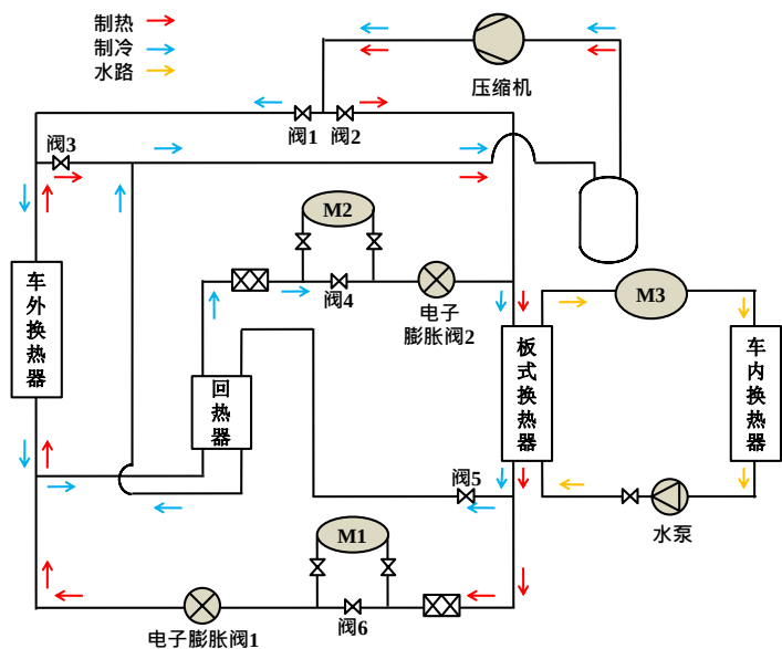
图 0-7 负荷侧采用二次换热回路的 R290 热泵系统
