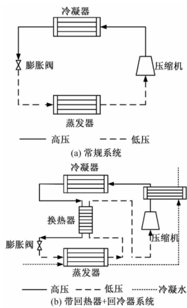
图 0-2 电动汽车空调系统循环原理 [238]
