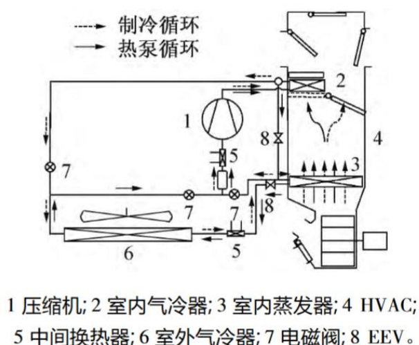
图 0-5 采用串联气冷器的 CO 2 车用热泵空调系统
