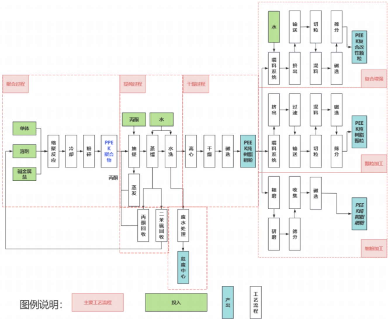
图表11: PEEK生产流程
