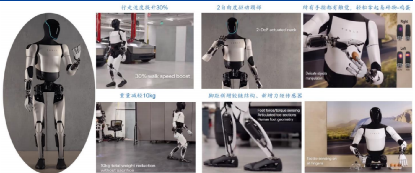
图表3：2023年12月特斯拉发布Optimus Gen-2
