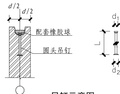
吊钉示意图
