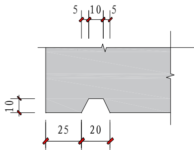
A7 滴水线做法
