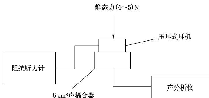
图6 压耳式耳机声反射纯音刺激信号声压级和总谐波失真的测量示意图
