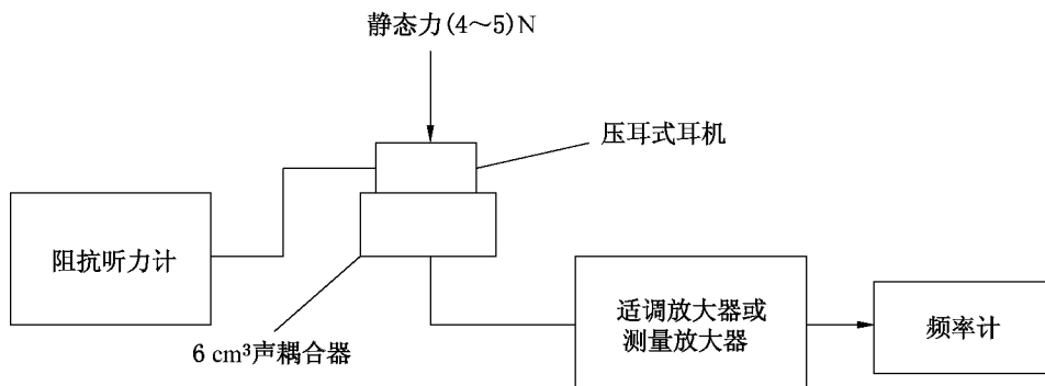
图5 压耳式耳机声反射纯音刺激信号频率的测量示意图
