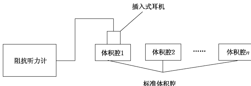
图 3 腔体积示值误差的测量示意图
