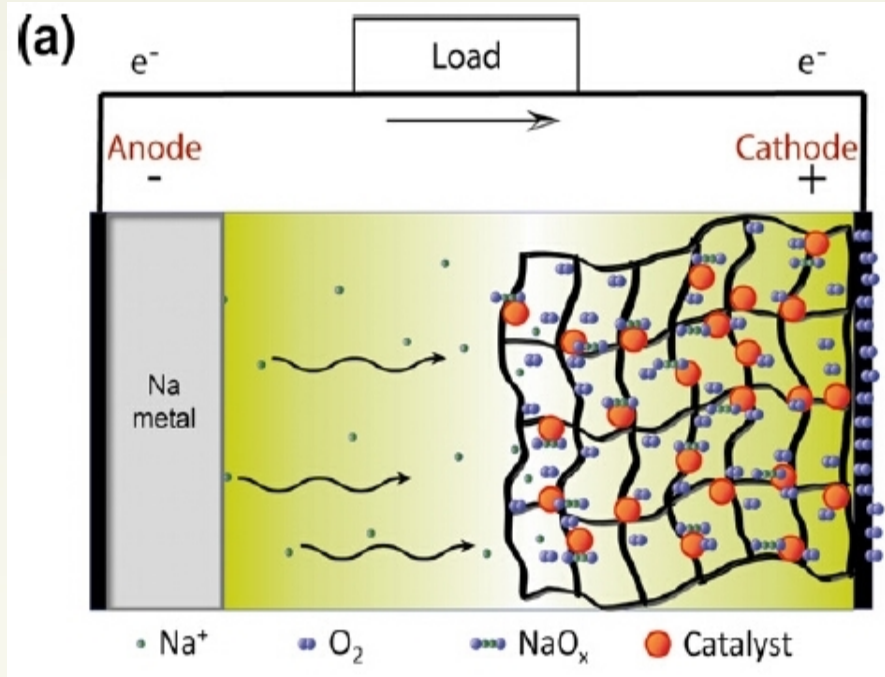
放电原理图
