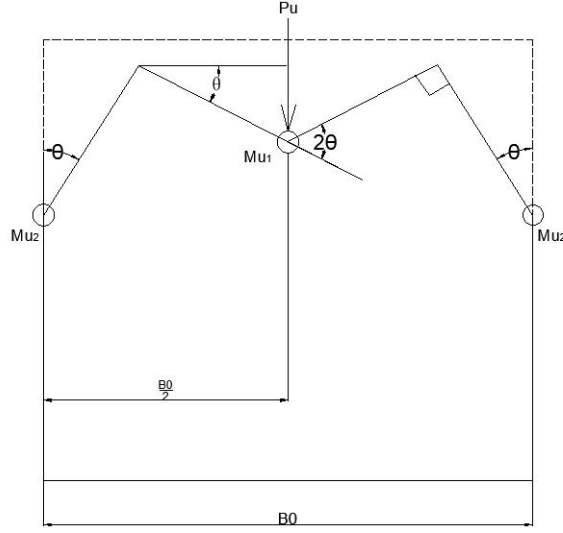
图 5.3.2-2 矩形管道受力状态示意图
