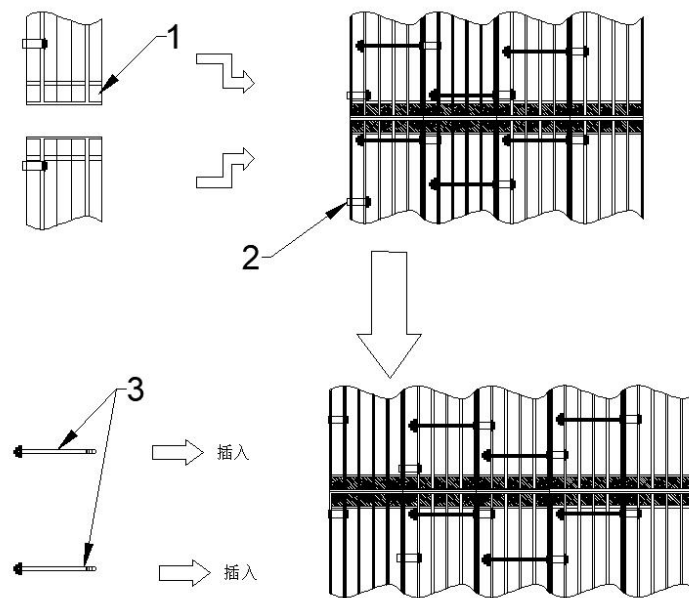
图 5.4.2-1 圆形管道纵向连接示意图
