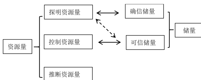
图A.1 资源量和储量类型及转换关系示意图
