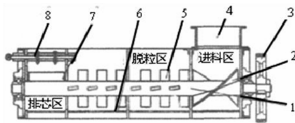
1 脱粒滚筒 2 入料区螺旋叶片 3V 带轮 4 入料斗 5 脱粒区板齿 6 栅格凹板 7 排芯区直板齿 8 排芯区压板机构
