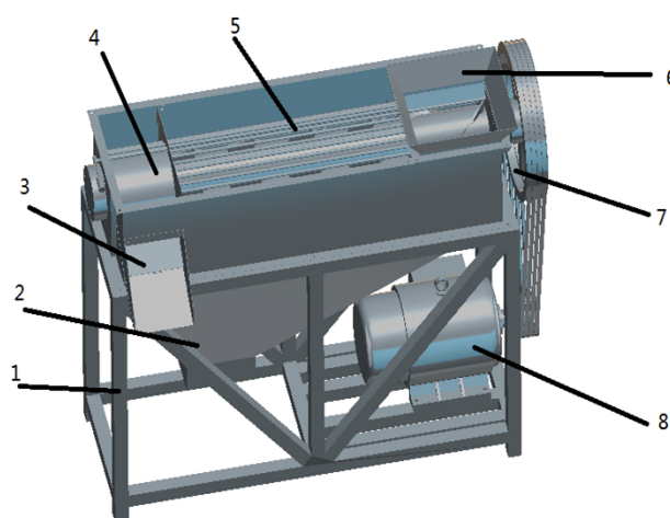
1 机架 2 出料口 3 排芯口 4 出料口压板 5 栅格凹板 6 入料口 7 带轮 8 电机
