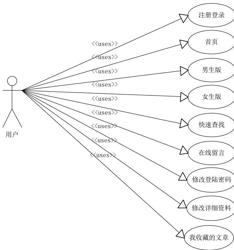
图 3-4 用户用例图
