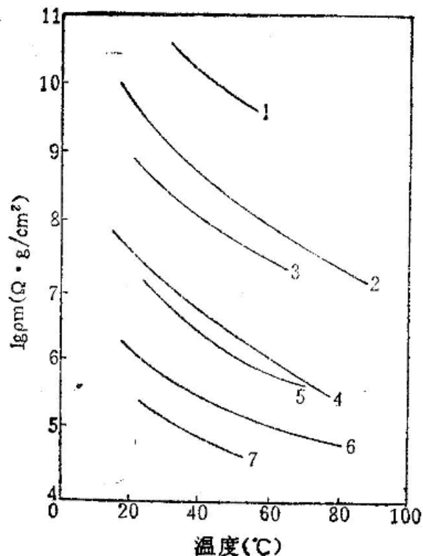
图 9-14 不同纤维的质量比电阻与温度、回潮率的关系 1—涤纶, W0.4% 2—锦纶, W6% 3—醋酯, W11.2% 4—羊毛, W15.4% 5—蚕丝, W14% 6—粘胶, W14.4% 7—棉, W9.9%
