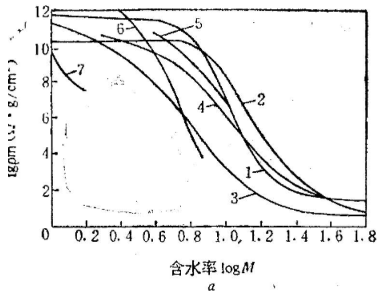
图 9-13 回潮率和相对湿度对质量比电阻的影响 a—含水率对质量比电阻的影响 b—相对湿度对质量比电阻的影响 1—蚕丝 2—羊毛 3—棉 4—粘胶 5—醋酯 6—锦纶 7— 8—涤纶
