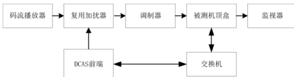
图1 可下载条件接收测量框图
