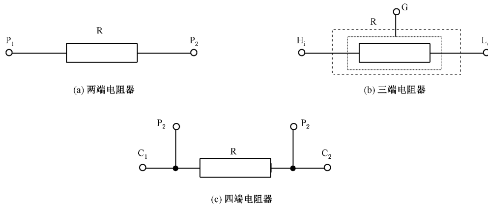
图 1 直流标准电阻器结构图
