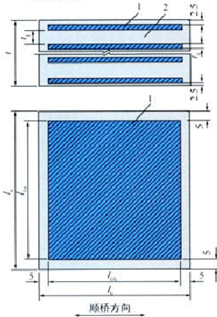
图1 矩形板式橡胶支座结构示意图（尺寸单位：mm） 1— 加劲钢板；2— 橡胶层
