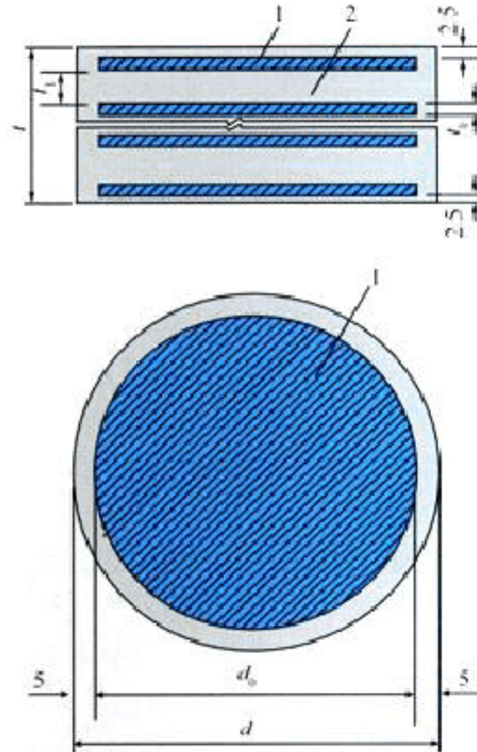
图2 圆形板式橡胶支座结构示意图（尺寸单位：mm） 1— 加劲钢板；2— 橡胶层
