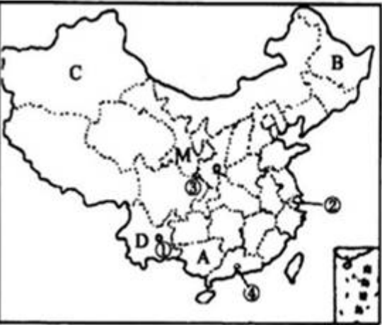
中国政区图
