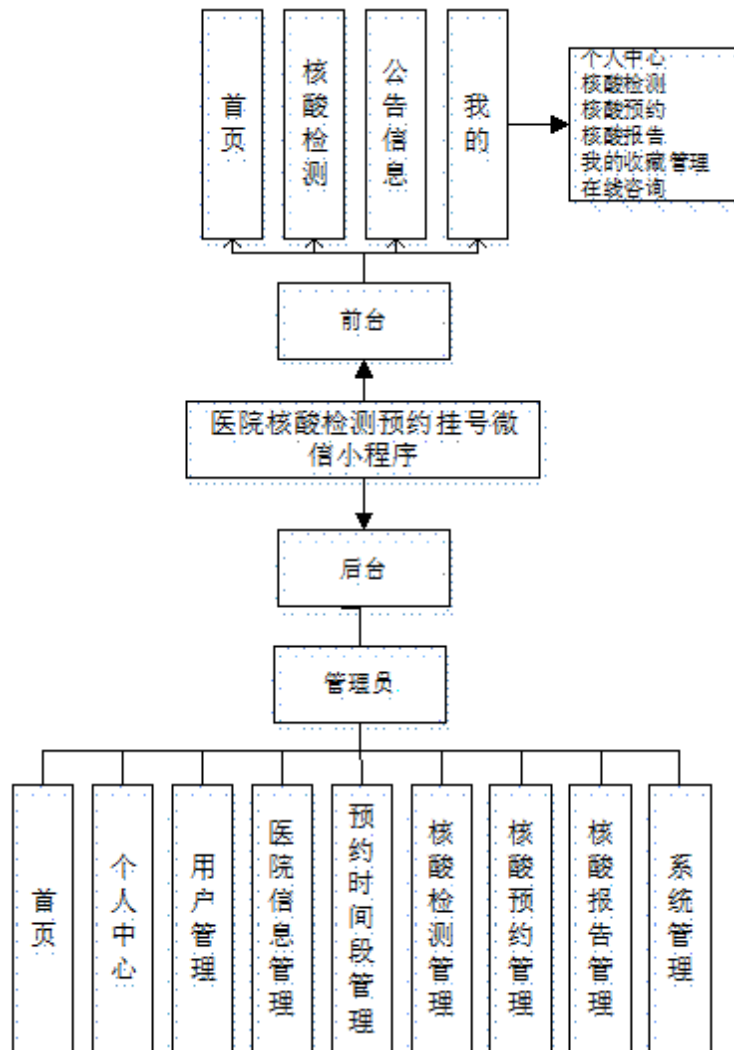
图 4-1 系统总体结构图
