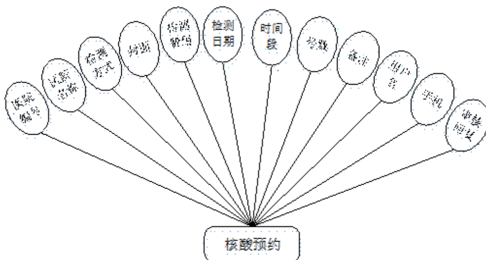
图 4-3 核酸预约 E/R 图
