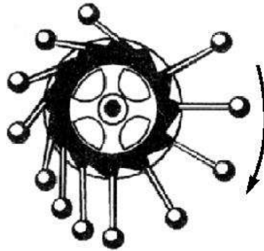
能量守恒和转化定律
