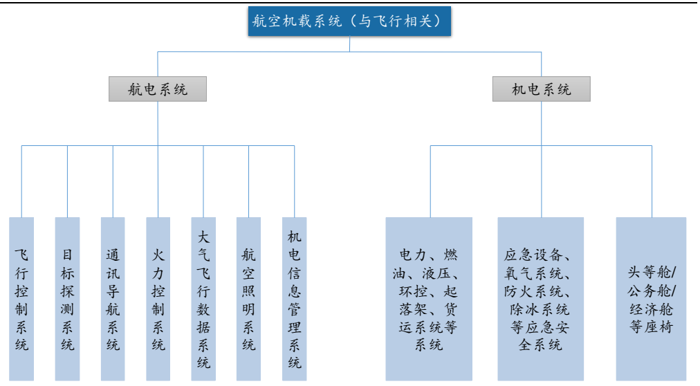
图 1：航空机载系统（与飞行相关）的构成
