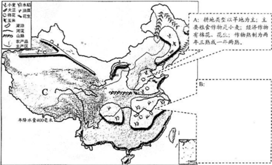
中国“十二五”规划农业战略格局示意图
