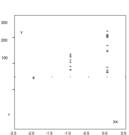
Y, X4 散点图
