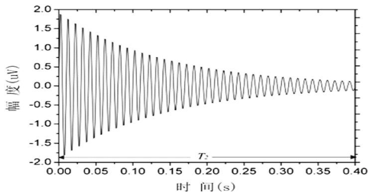
图A.3 拉莫尔进动产生的自由感应衰减信号(FID)示意图
