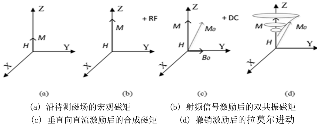
图A.2 欧弗豪泽传感器的工作过程示意图
