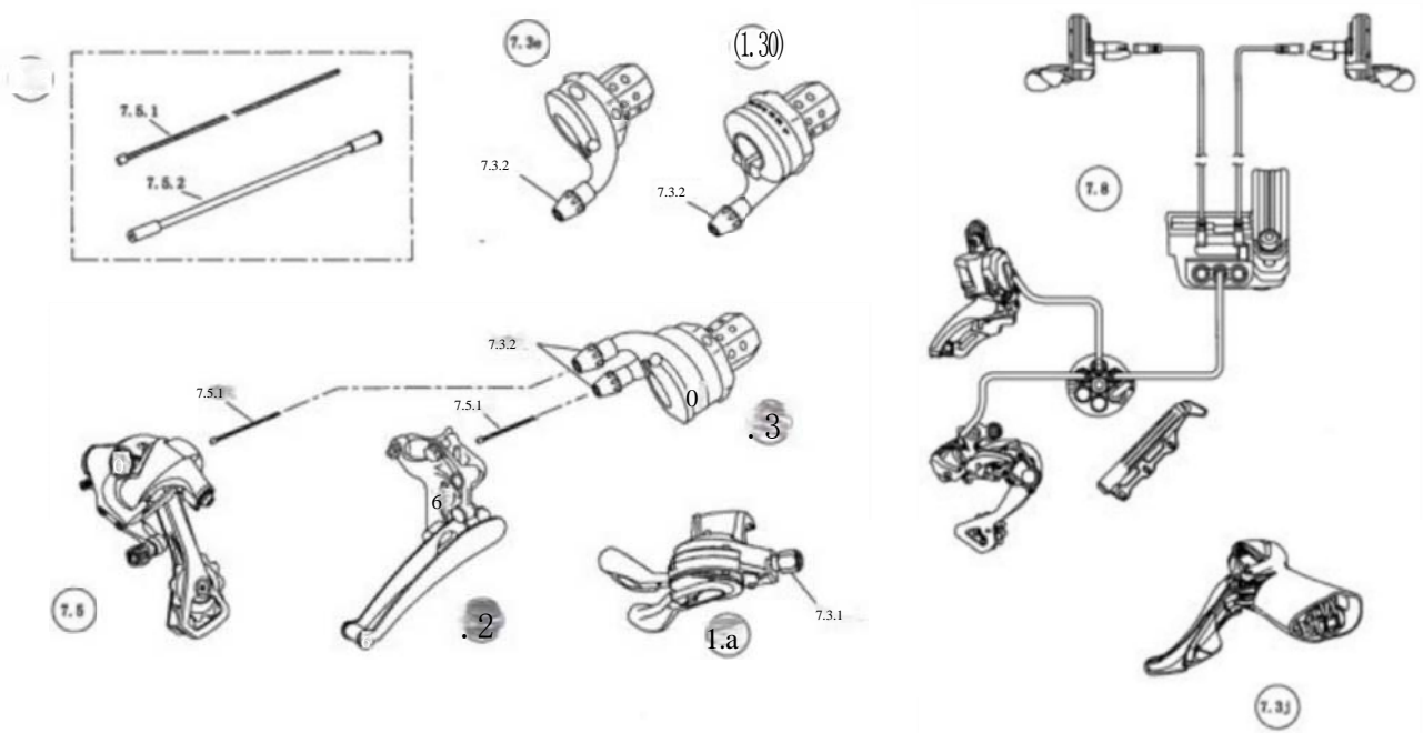
图 1 4 拔链器部件 (2)
