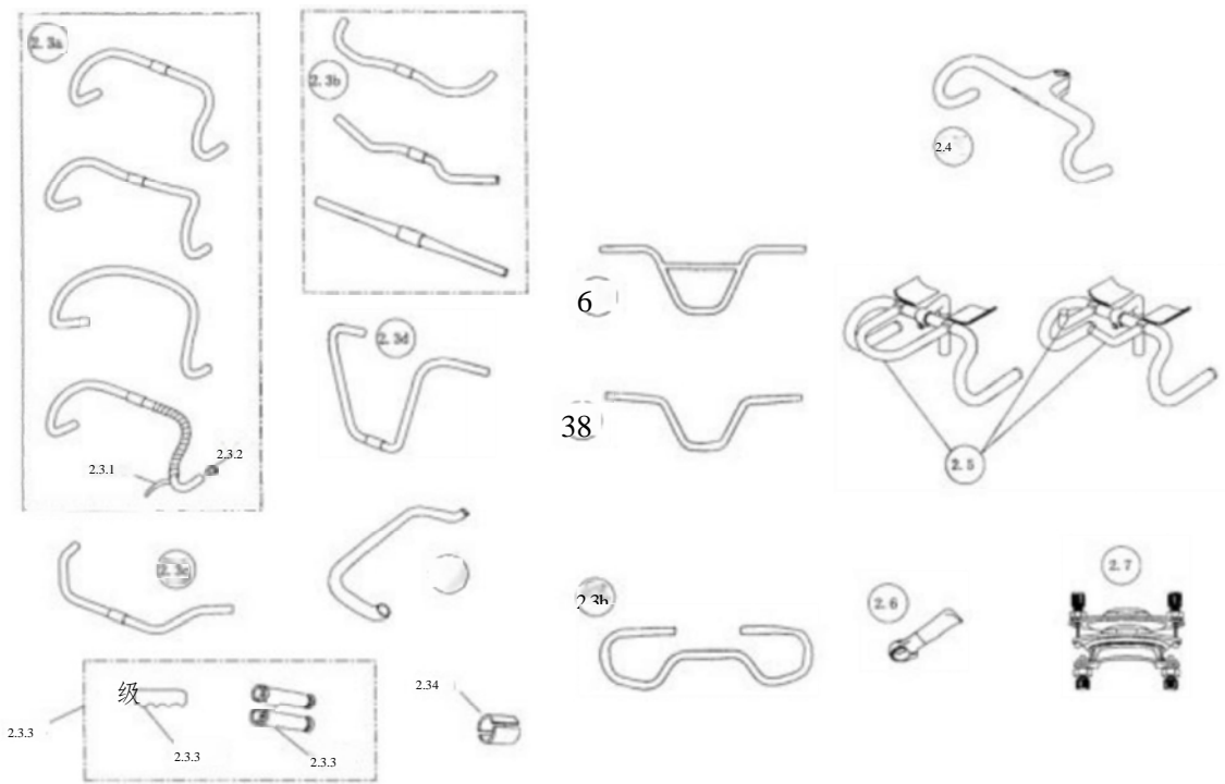
图 4 车头部件(2)
