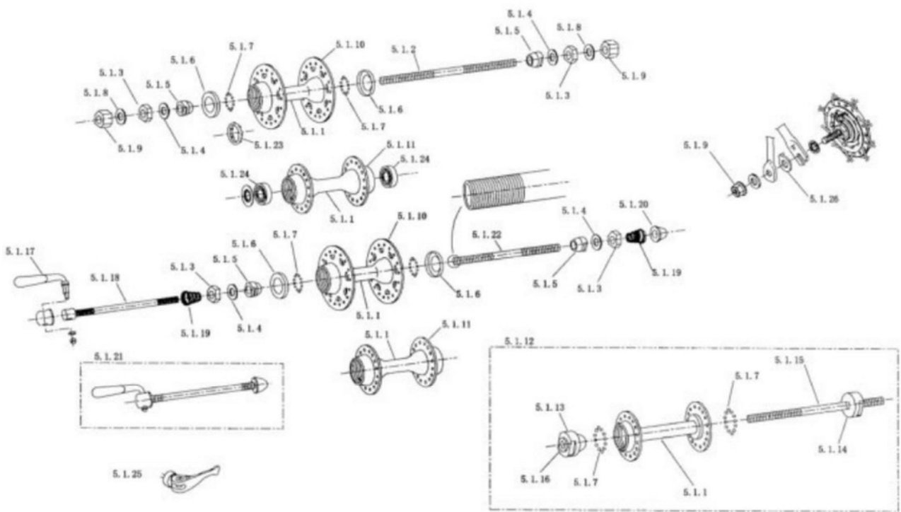
图10 前轴部件(2)
