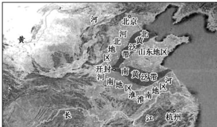
黄泛区示意图
