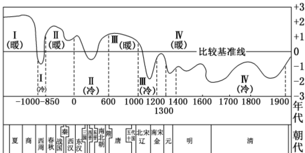
中国古代气温变化曲线图
