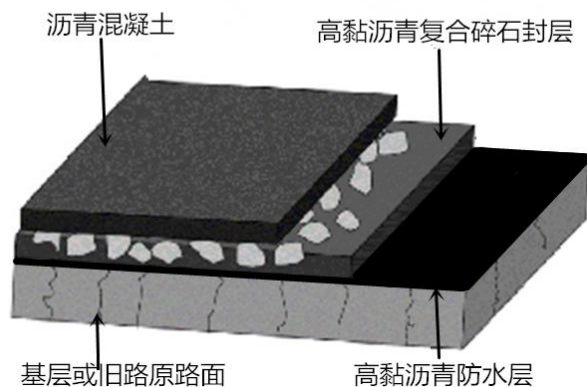
图 1 公路高黏沥青复合碎石封层结构层位示意图
