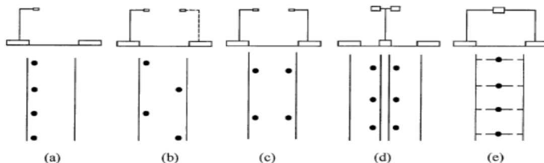
图1 常规照明灯具布置的五种基本方式
