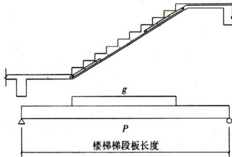
图 14-3-2 折板楼梯梯段板配筋简图
