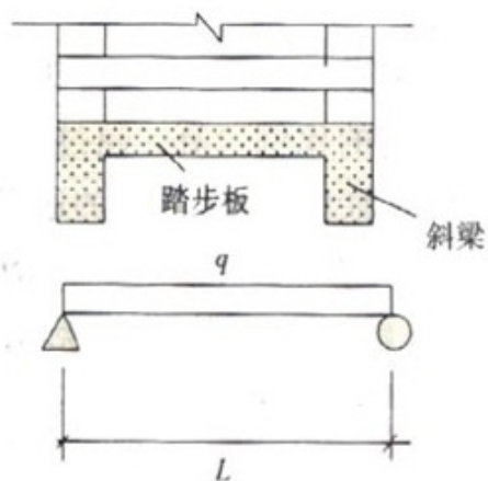
图 14-2-2 踏步板计算简图
