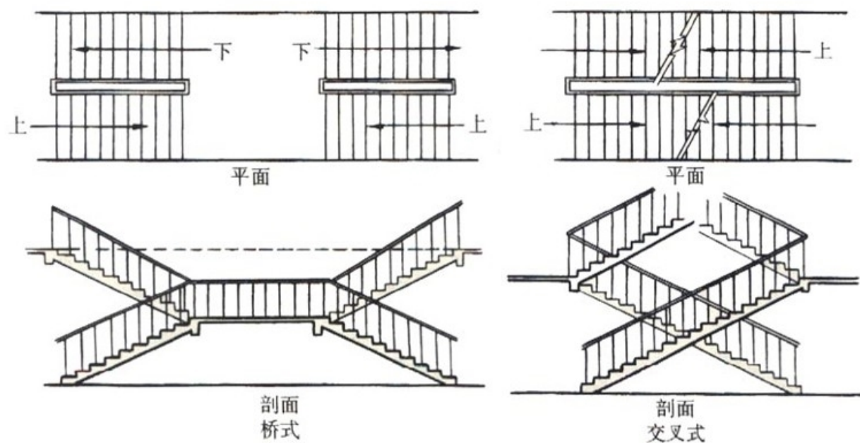
图14-1-1 楼梯形式之二
