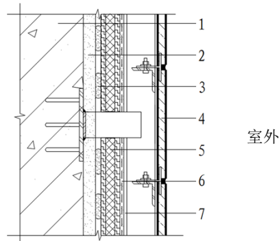
1—基层墙体；2—防水层；3—粘结层；4—非透明幕墙；5—套装双真空保温隔热板； 6—抹面层（内嵌玻纤网）；7—饰面层
