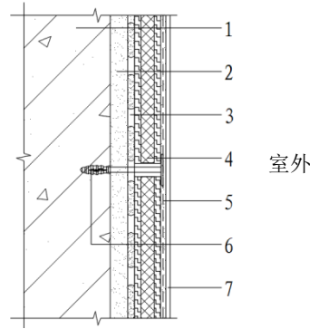
1—基层墙体；2—防水层；3—粘结层；4—套装双真空保温隔热板；5—抹面层（内嵌玻纤网）； 6—锚栓；7—饰面层
