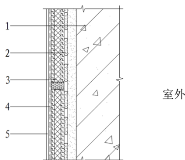
1—基层墙体；2—粘结层；3—套装双真空保温隔热板；4—抹面层（内嵌玻纤网）；5—饰面层
