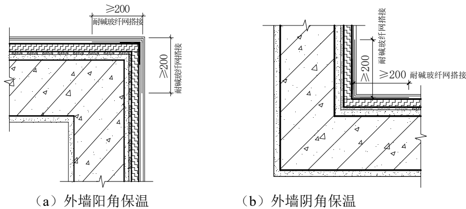
图 5.3.7 外墙阳角、阴角保温
