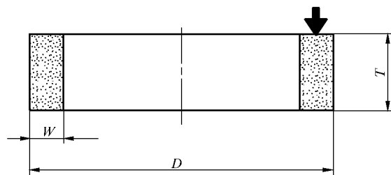
图 1 2 型砂轮
