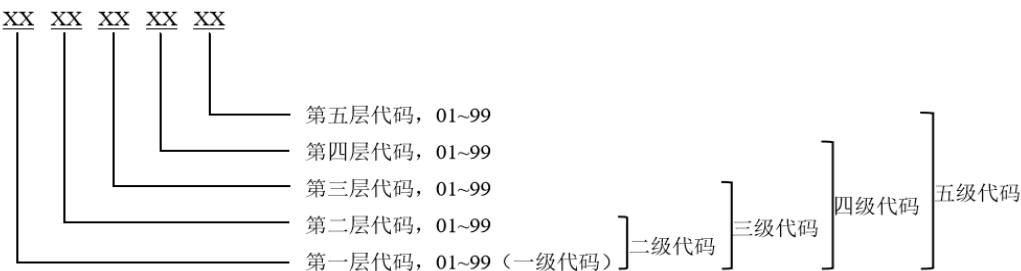
图1 代码结构图
