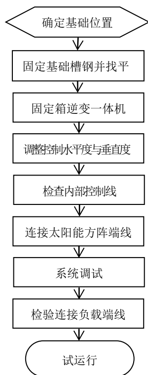
图 7.3.3 箱逆变一体机安装流程图
