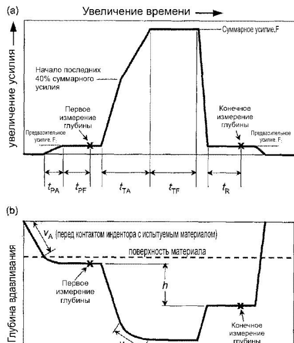
Рис. 2 Схематические диаграммы "усилие – время" (а) и "глубина индентора – время" (б) испытания HRC, демонстрирующие части цикла испытаний
