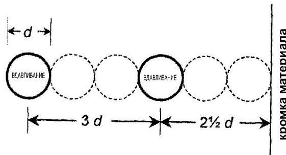
РИС. 3. Схема минимального пространства для вдавливания
