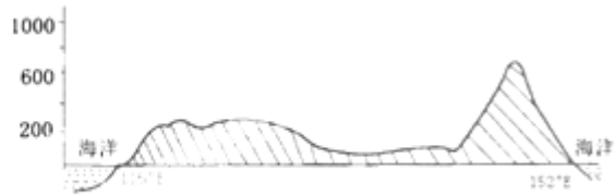
澳大利亚沿30° S地形剖面图
