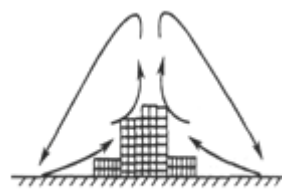
某城市“热岛效应”
