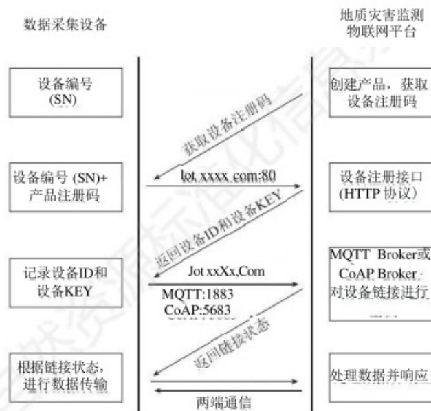
图 7 数据采集设备注册连接步骤示意图
