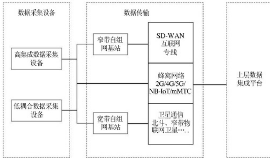
图 1 地质灾害监测通信总体架构示意图
