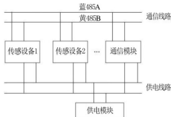
图 4 传感设备与通信模块的接口示意图
