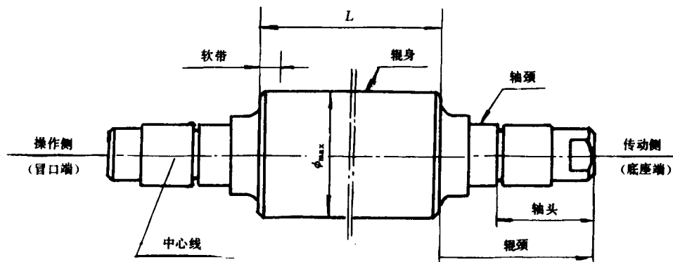
轧辊示意图
