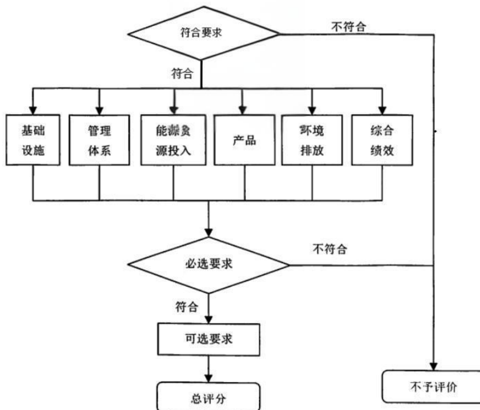
绿色电厂评价流程
