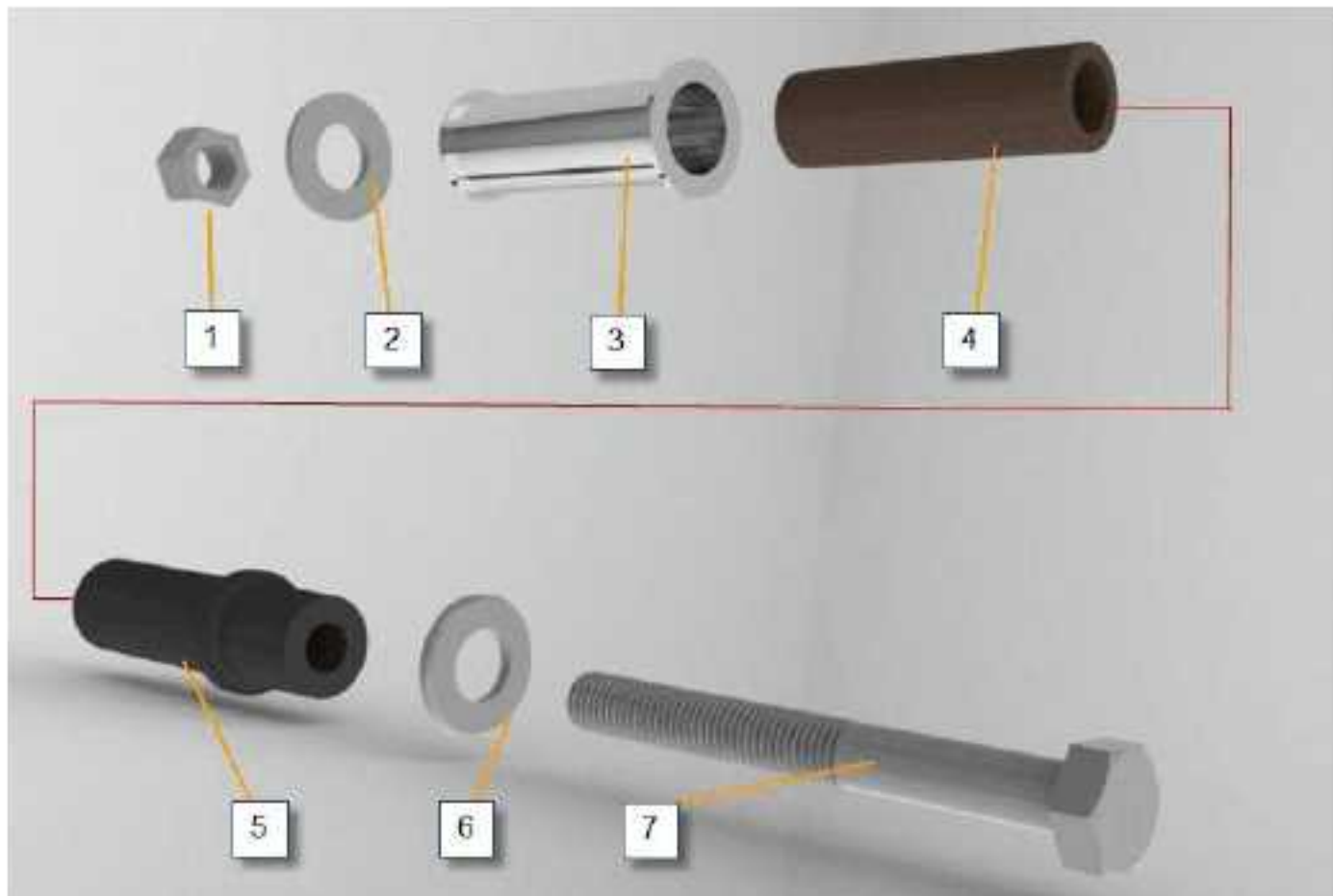
图 3-6 导向销装配
