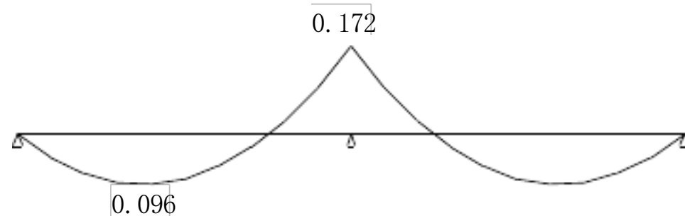
计算简图
