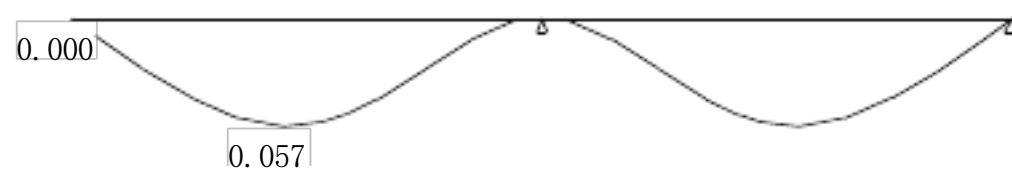
支撑钢管变形图(mm)
