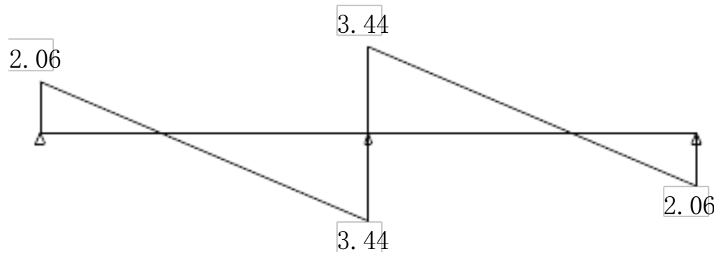
剪力图(kN)
