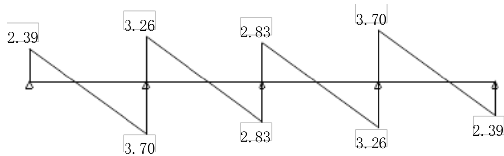
剪力图(kN)
