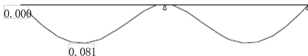
变形图(mm)
