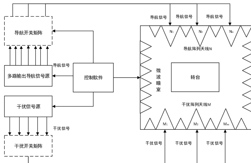
图 1 满天星导航测试系统原理图
