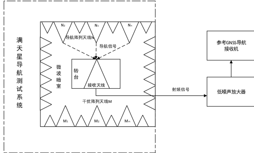
图 7 满天星定位偏差校准
