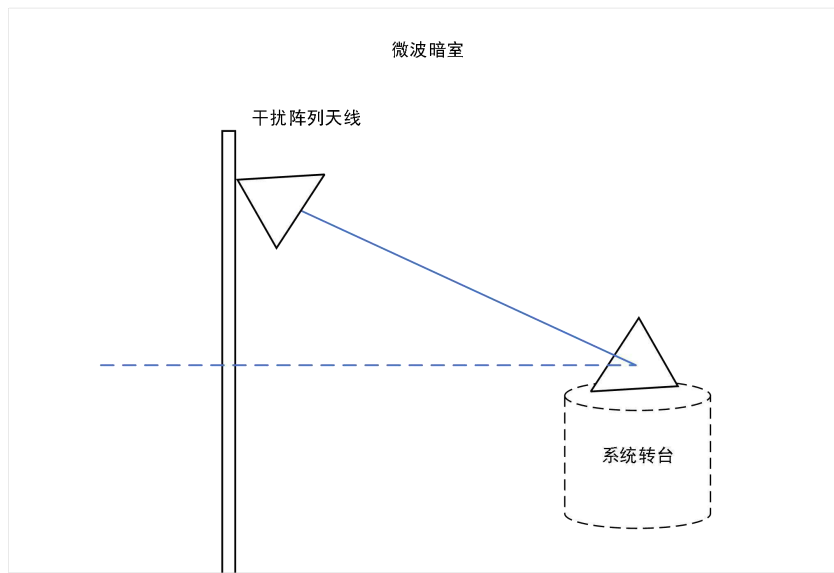
图 6 干扰来向角度校准
