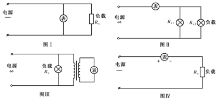
电压、电流表测量接线图（多组）示意图
