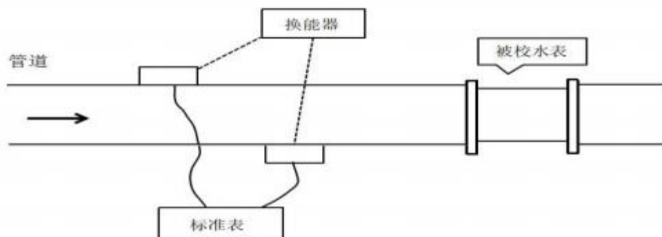
图 1 标准表安装示意图
