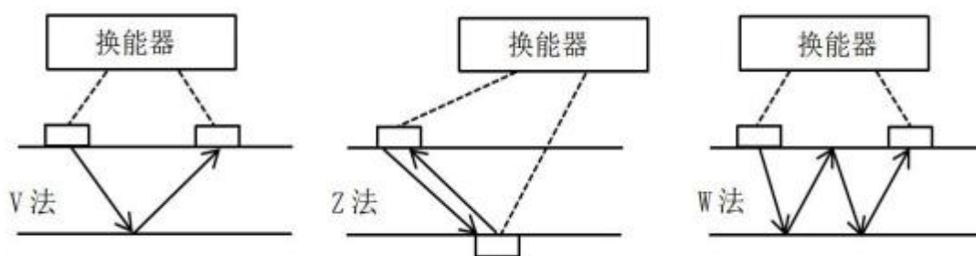
图 2 换能器安装方式示意图
