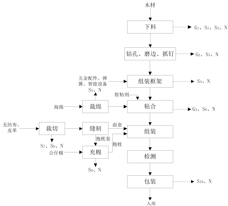
图 2-3 智能家居生产工艺流程及产污环节图
