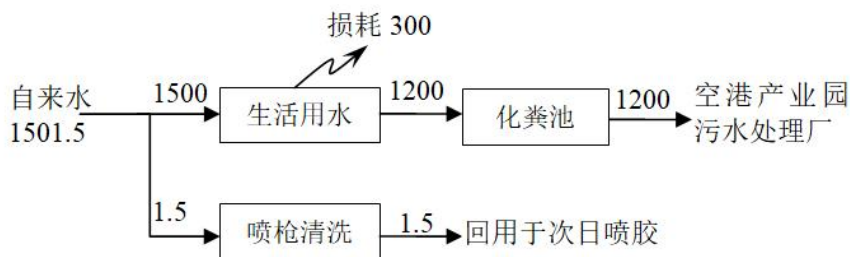
图 2-1 本项目水平衡图 (单位: t/a)
