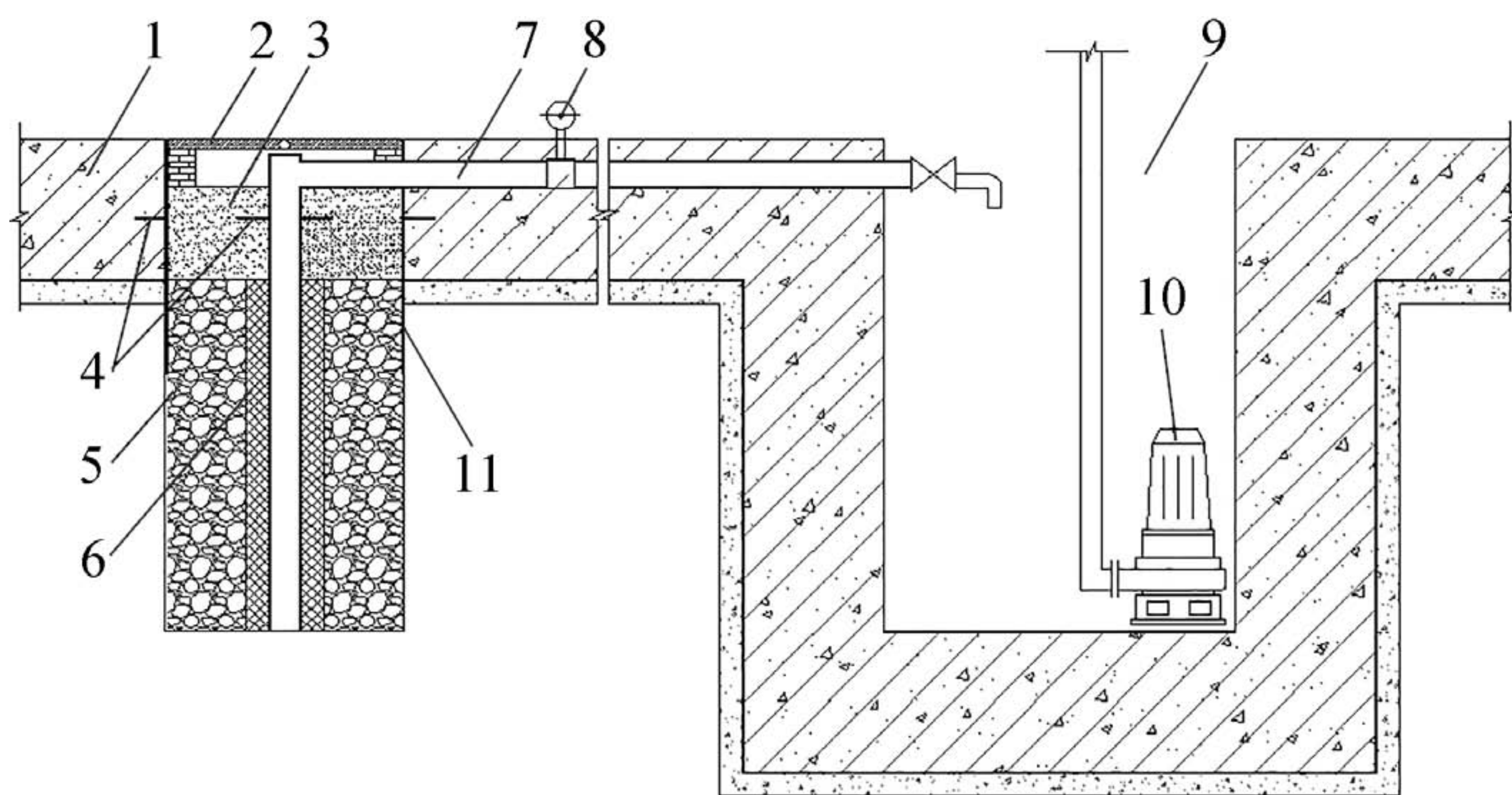
1—基础底板;2—井盖;3—封孔灌浆料;4—止水材料;5—反滤层;6—过滤装置; 7—导水管;8—减压球阀;9—集水坑;10—抽水泵;11—钢护筒
