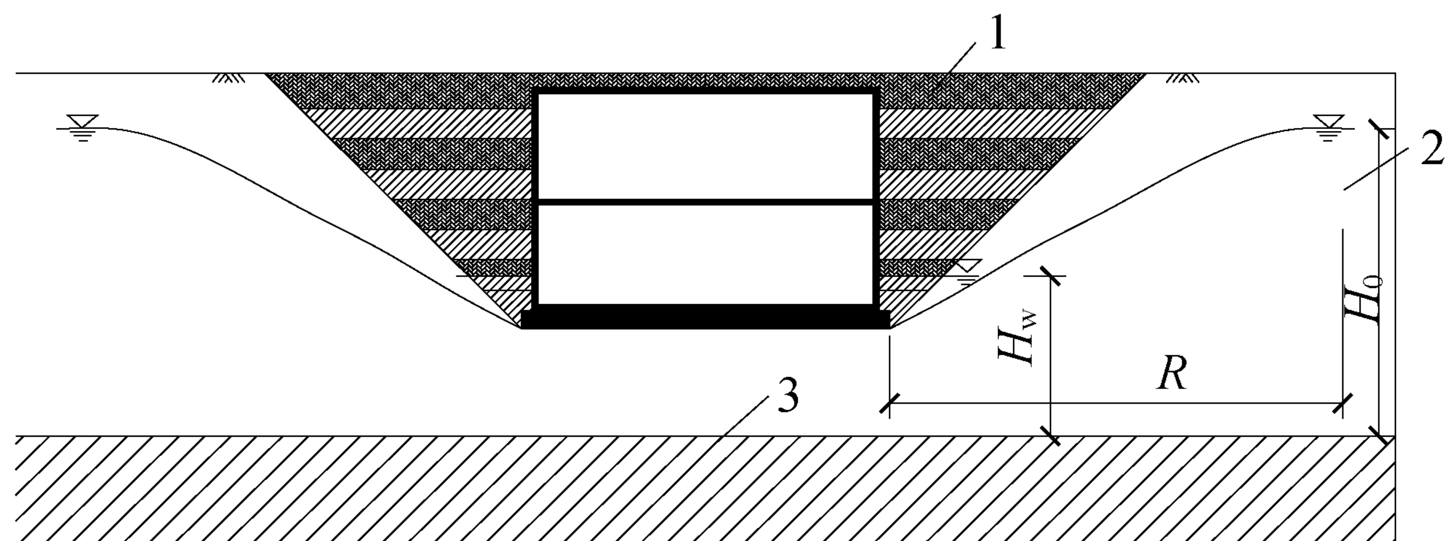
1—肥槽; 2—潜水含水层; 3—弱透水性土层
