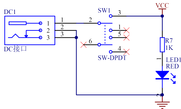
图 3 电源电路
