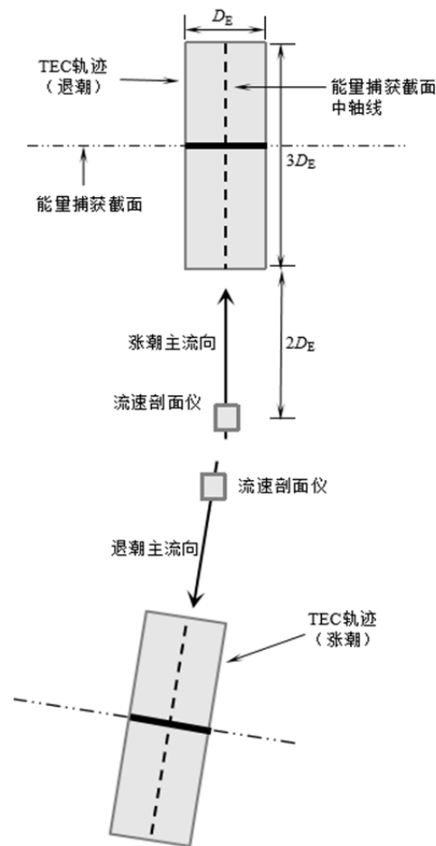
图 5 漂浮式装置流速测试仪器的布放（俯视图）
