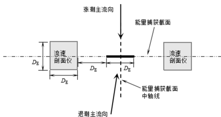
图3 方案二 测量仪器的两侧布放（俯视图）
