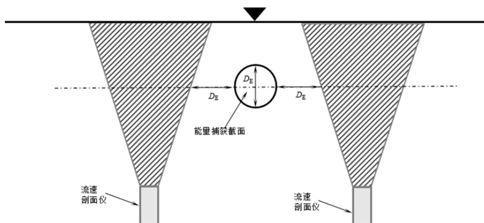
图4 方案二 测量仪器的两侧布放（剖视图）
