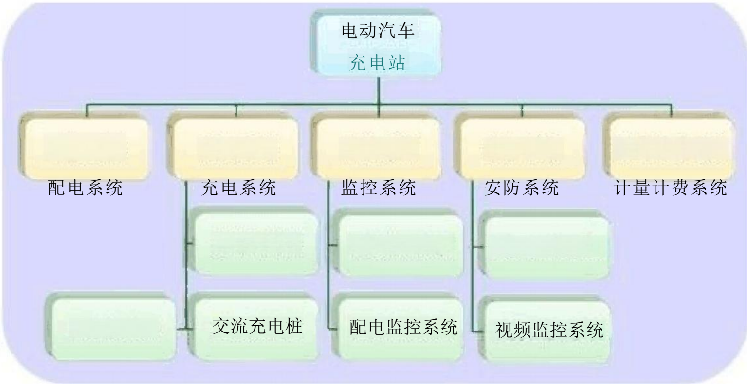
电动汽车充电站系统框图
