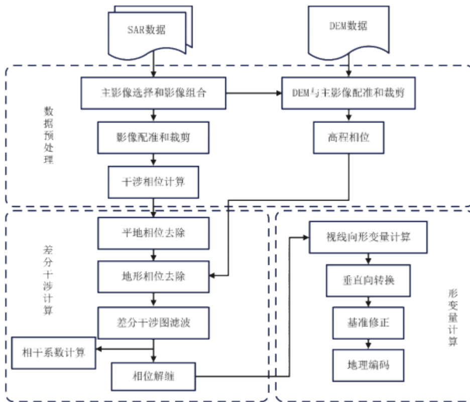
图2 D-InSAR 数据处理流程图
