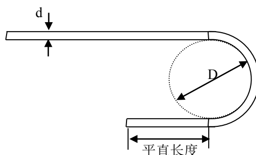
图 3-6 钢筋弯钩示意图
